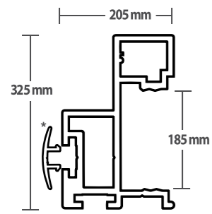
Άνω οδηγός διπλός
