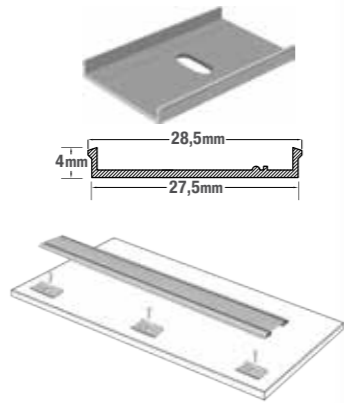
Κούμπωμα κάτω οδηγού
