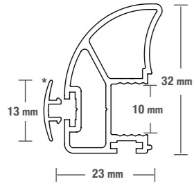
Άνω οδηγός διπλός
