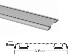
Κάτω οδηγός μονός
