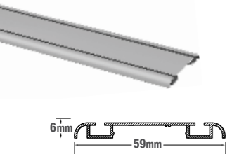
Κάτω οδηγός μονός
