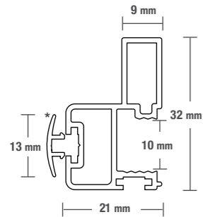
Άνω οδηγός διπλός
