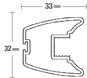
Άνω οδηγός διπλός
