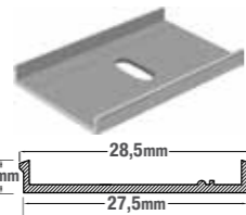
Κούμπωμα κάτω οδηγού
