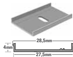
Κούμπωμα κάτω οδηγού
